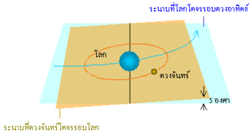
ภาพที่ 1 ระนาบวงโคจรของดวงจันทร์ ตัดกับ ระนาบวงโคจรของโลก เป็นมุม 5^{\circ}
