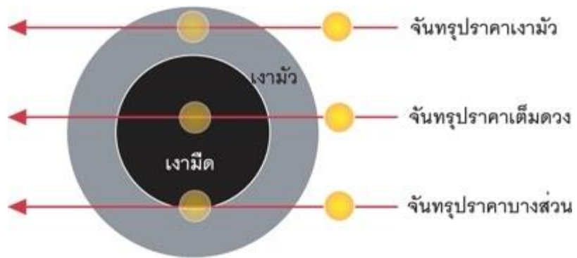
ภาพที่ 3 จันทรุปราคาชนิดต่างๆ
